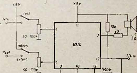
Fig. 2. Signalering met regelbaar referentie niveau.
